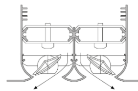
LANCIO ORIZZONTALE 2 DIREZIONI TWO DIRECTION HORIZONTAL THROW
