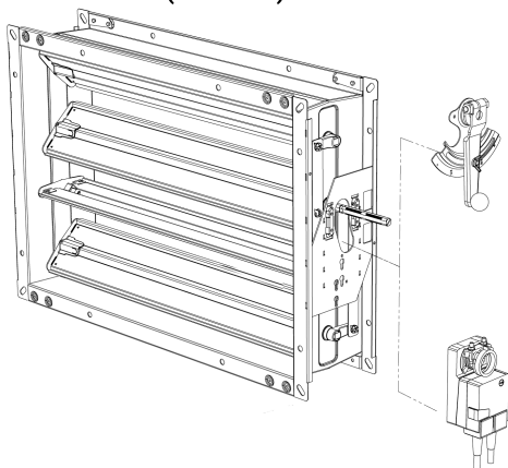
Perno e piastra universale (standard)
