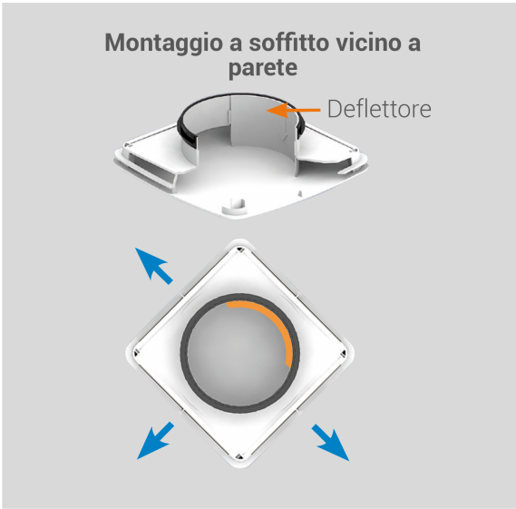
Montaggio a parete o soffitto
