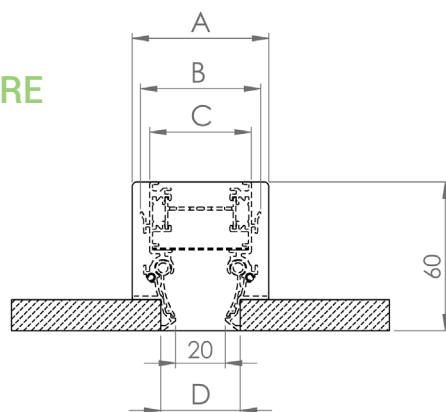
EDLH-FA 1 feritoia 20 mm EDLHB-FA 1 feritoia 20 mm
