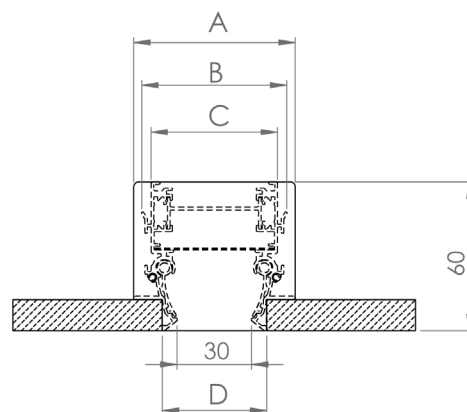
EDLH-FB 1 feritoia 30 mm EDLHB-FB 1 feritoia 30 mm
