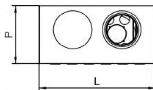
VISTA SUPERIORE PASSAGGI PER ARIA EXT ed ESPULSIONE
