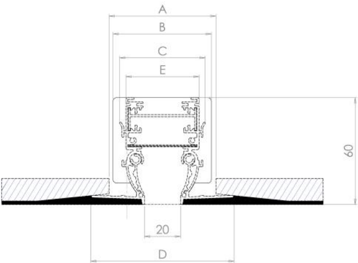
EDLS-FA 1 feritoia 20 mm EDLSB-FA 1 feritoia 20 mm
