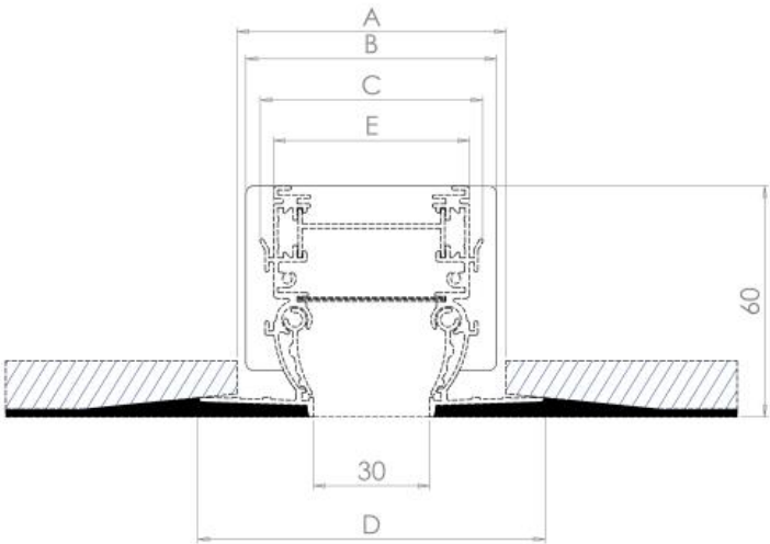
EDLS-FB 1 feritoia 30 mm EDLSB-FB 1 feritoia 30 mm
